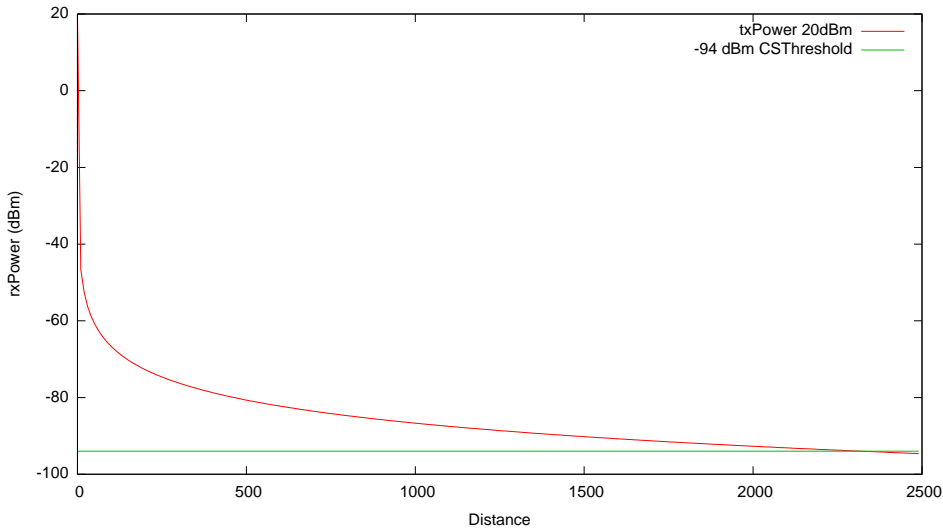
ns3::FriisPropagationLossModel (Default Parameters)
